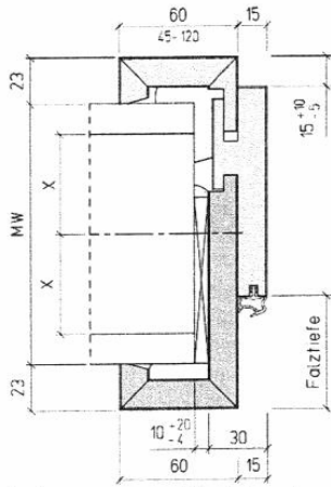
Holzfeuerzarge für Massivwand
