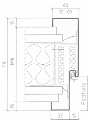
Stahlzarge für Leichtbauwand Hutankermontage
