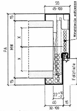
Stahlzarge für Massivwand 2-teilig, mit Laschen-Klemm-Befestigung
